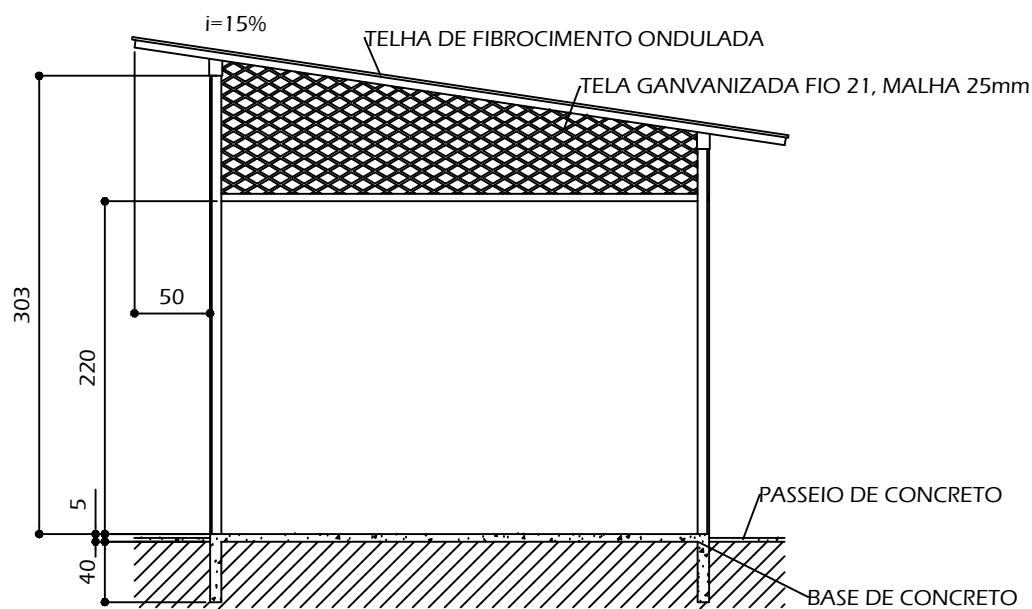
ELEVACÃO ESCALA 1/50
