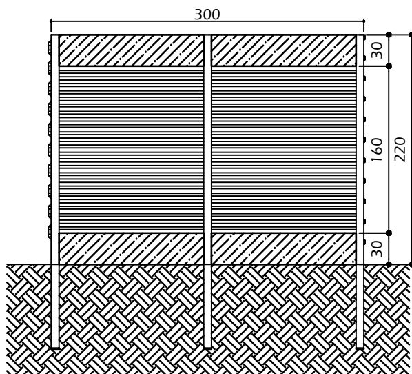
VISTA POSTERIOR ESCALA 1/50
