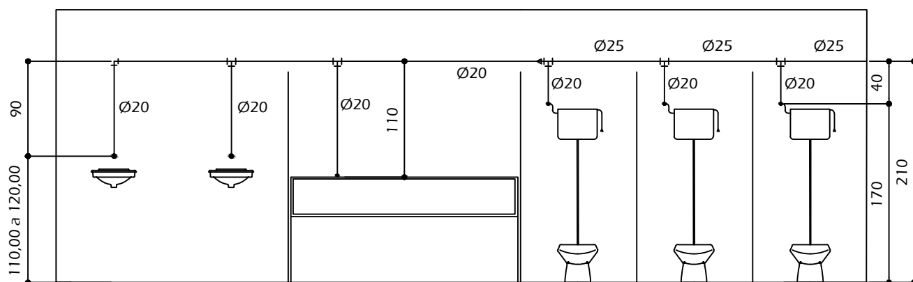
ÁGUA FRIA - PAREDE 1 - INSTALAÇÃO SANITÁRIA TIPO III ESCALA 1/50
