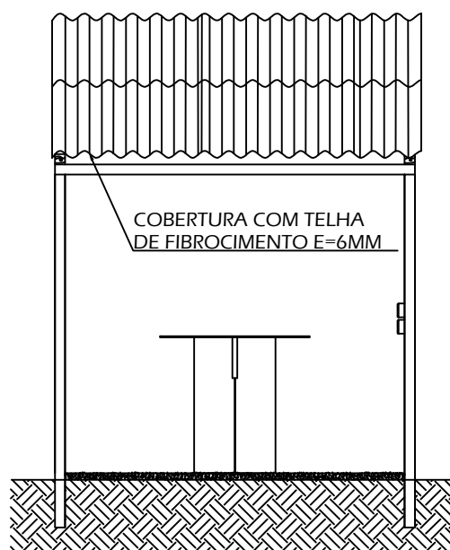
ELEVAÇÃO FRONTAL
