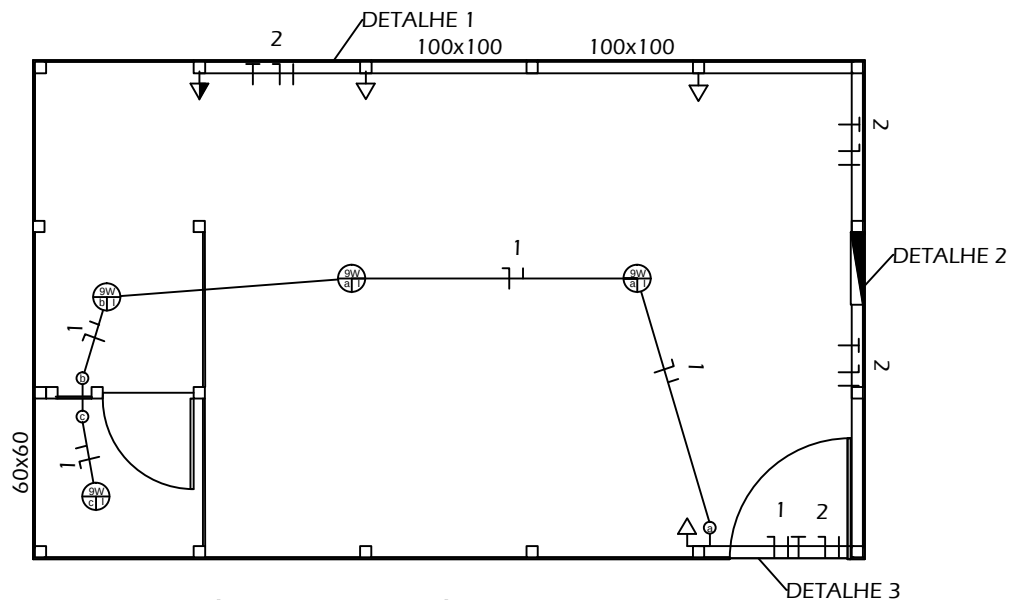
PLANTA - ELÉTRICO ESCRITÓRIO TIPO I
