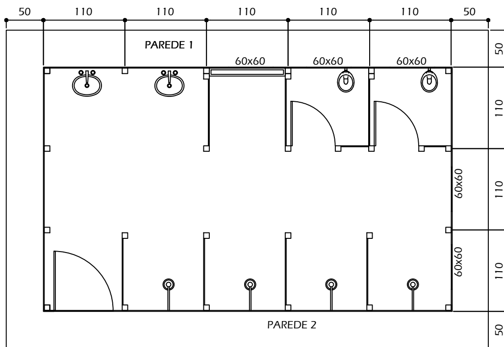
PLANTA - INSTALAÇÃO SANITÁRIA TIPO II
