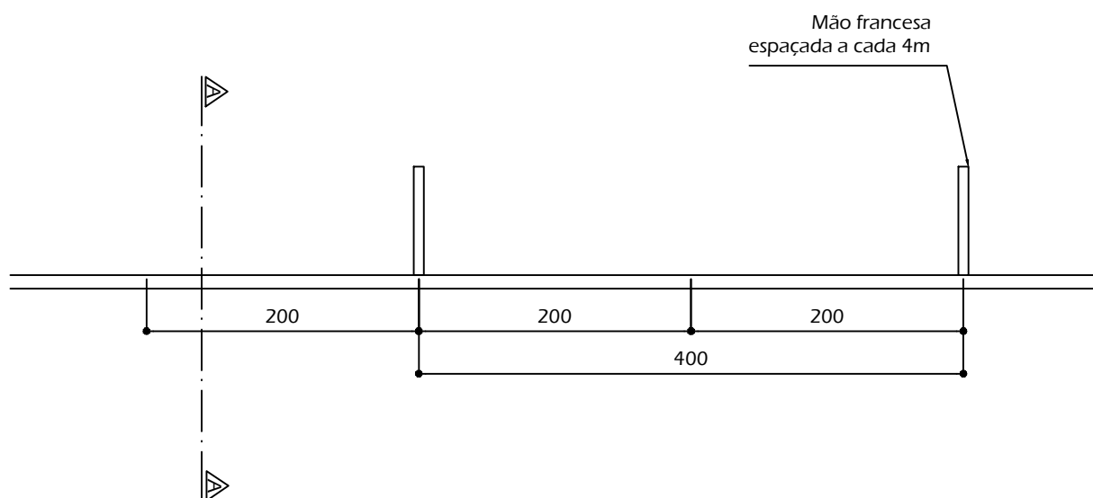
PLANTA ESCALA 1/50
