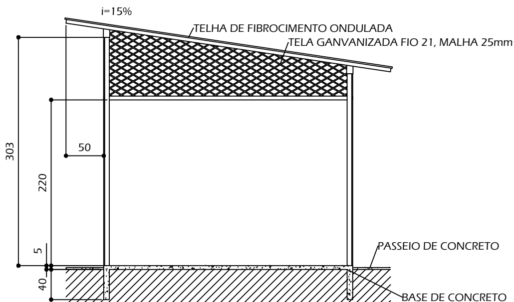
ELEVAÇÃO ESCALA 1/50
