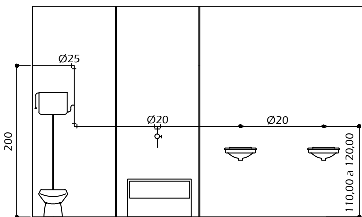
ÁGUA FRIA - PAREDE 1 - INSTALAÇÃO SANITÁRIA TIPO I
