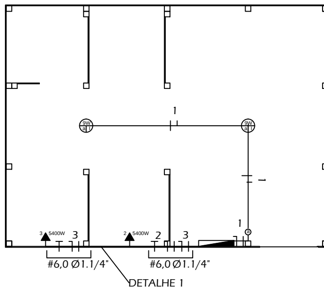
PLANTA - ELÉTRICO INSTALAÇÃO SANITÁRIA TIPO I
