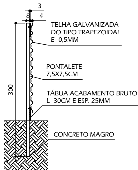
ELEVAÇÃO LATERAL ESCALA 1/50
