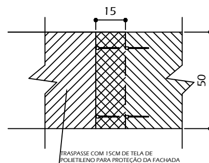
DETALHE 3 ESCALA 1/20
