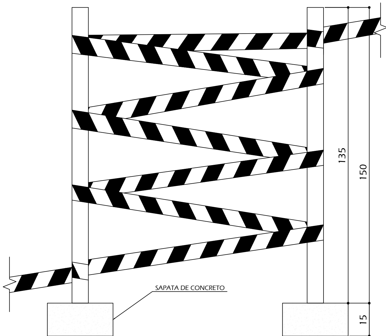
ELEVAÇÃO ESCALA 1/10
