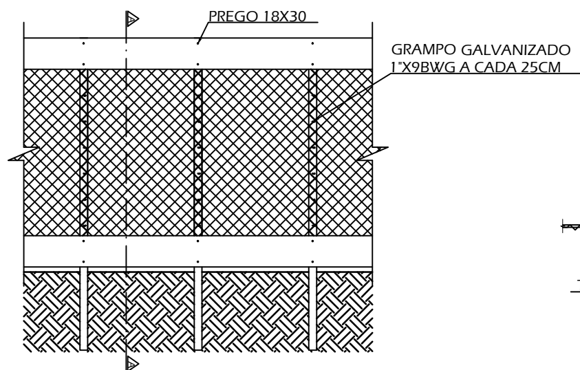
ELEVAÇÃO FRONTAL ESCALA 1/50
