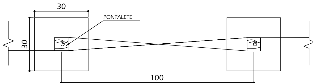
PLANTA ESCALA 1/10
