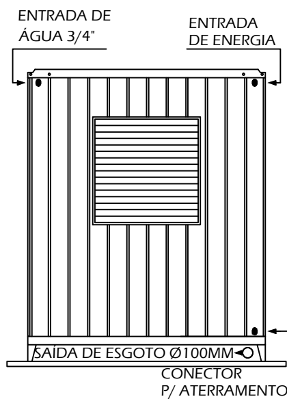
VISTA POSTERIOR ESCALA 1/50
