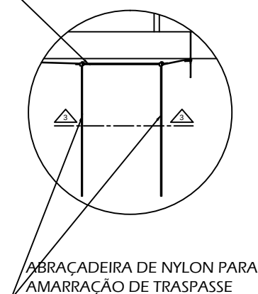
DETALHE 2 ESCALA 1/10
