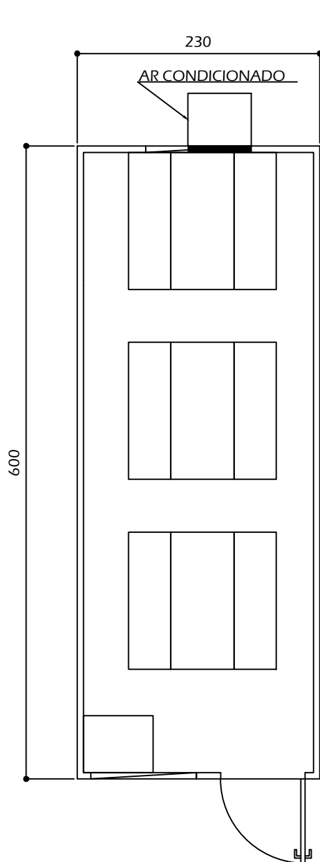
PLANTA ESCALA 1/50
