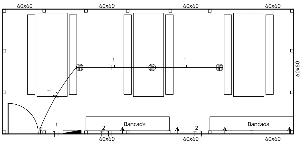
PLANTA - ELÉTRICO REFEITÓRIO TIPO II
