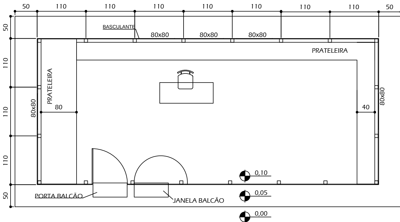
PLANTA - DEPÓSITO DE FERRAMENTAS TIPO II ESCALA 1/50
