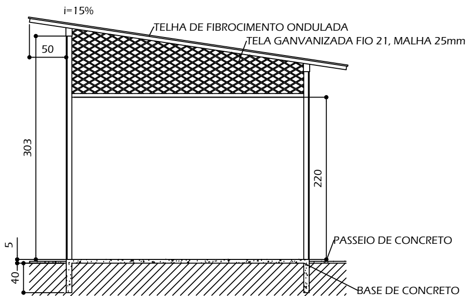
ELEVAÇÃO ESCALA 1/50
