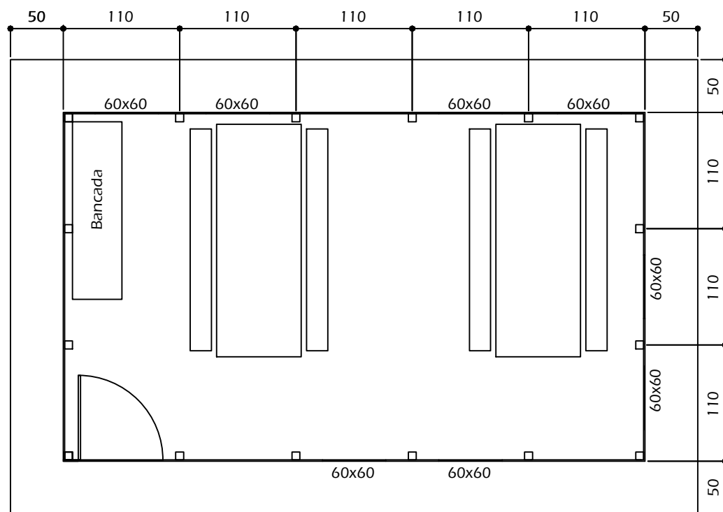
PLANTA - REFEITÓRIO TIPO I
