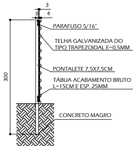
ELEVAÇÃO LATERAL ESCALA 1/50
