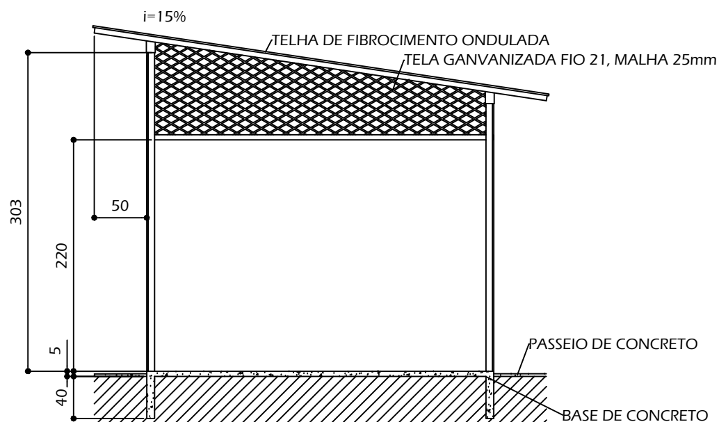
ELEVACÃO ESCALA 1/50
