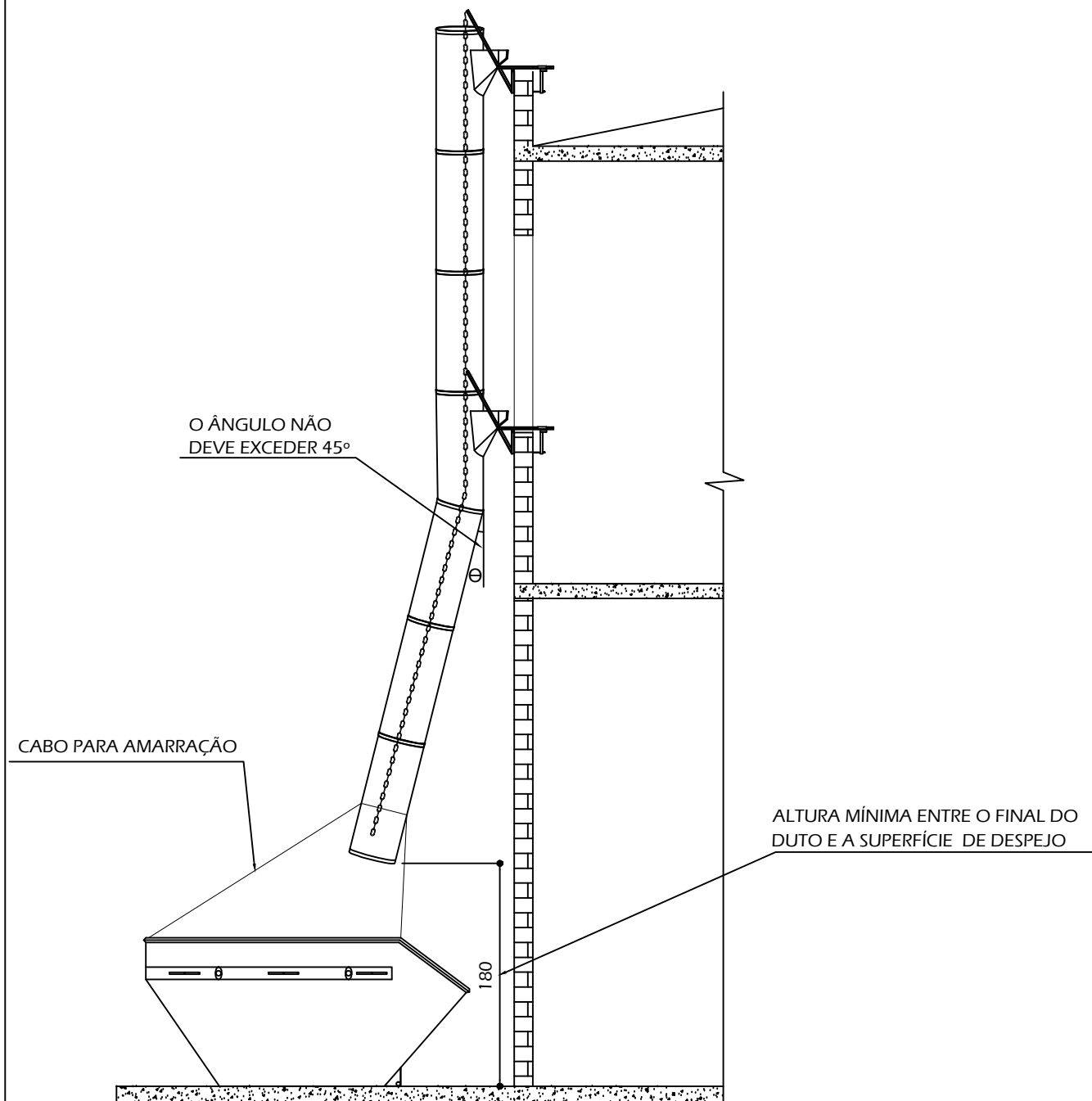
ELEVACÃO
