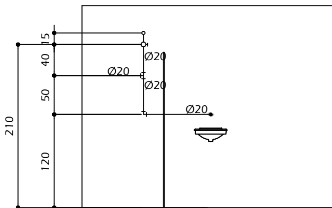
ÁGUA FRIA - PAREDE 1 - ESCRITÓRIO TIPO II
