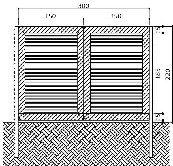
VISTA POSTERIOR ESCALA 1/50
