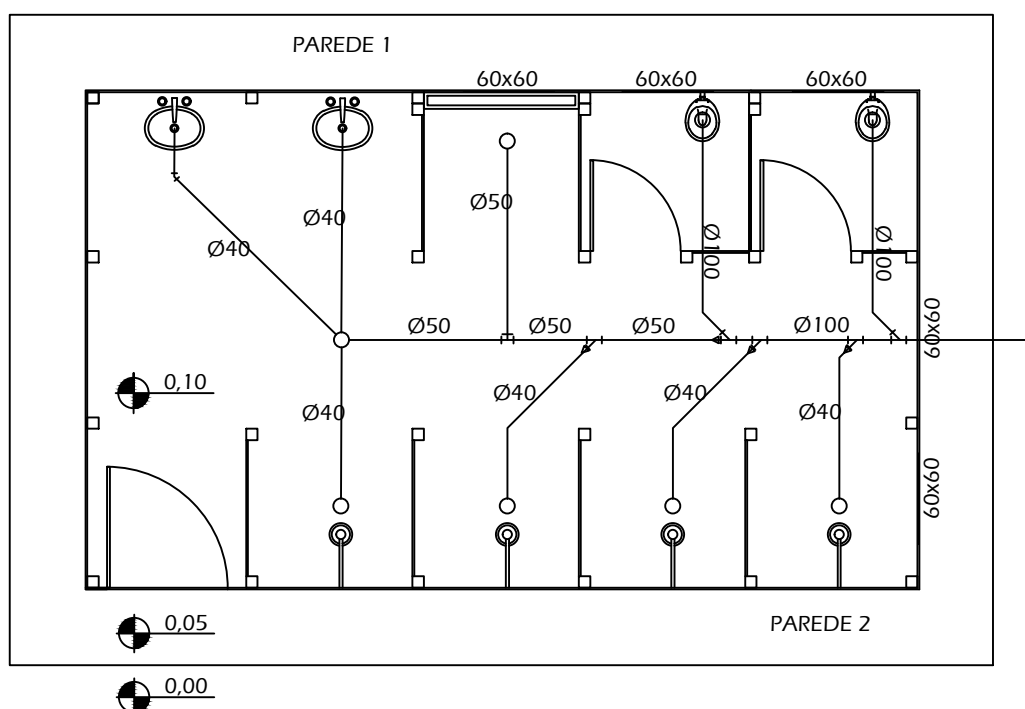
PLANTA SANITÁRIO - INSTALAÇÃO SANITÁRIA TIPO II
