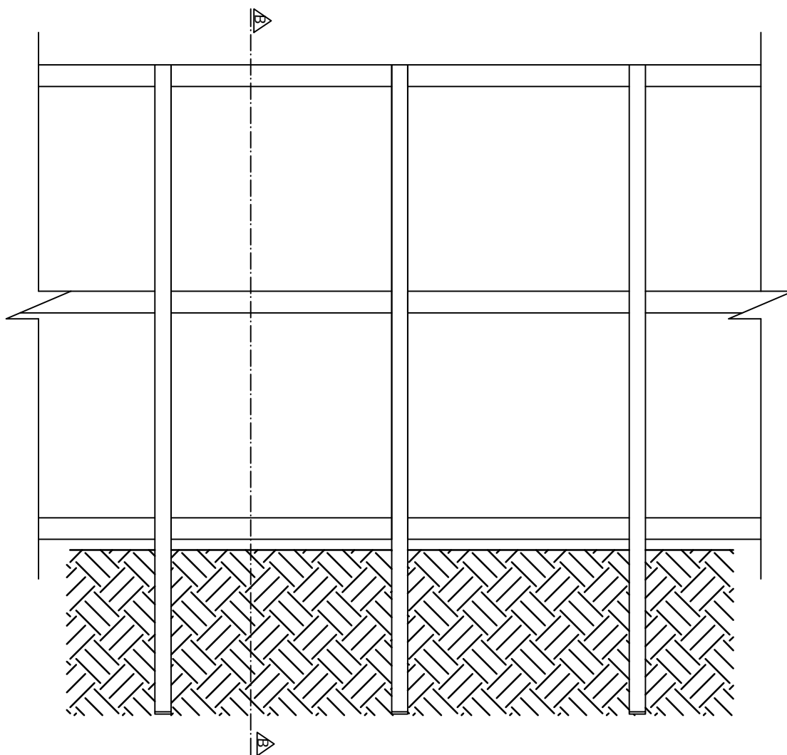
VISTA POSTERIOR ESCALA 1/25
