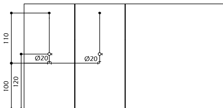
ÁGUA FRIA - PAREDE 2 - INSTALAÇÃO SANITÁRIA TIPO I
