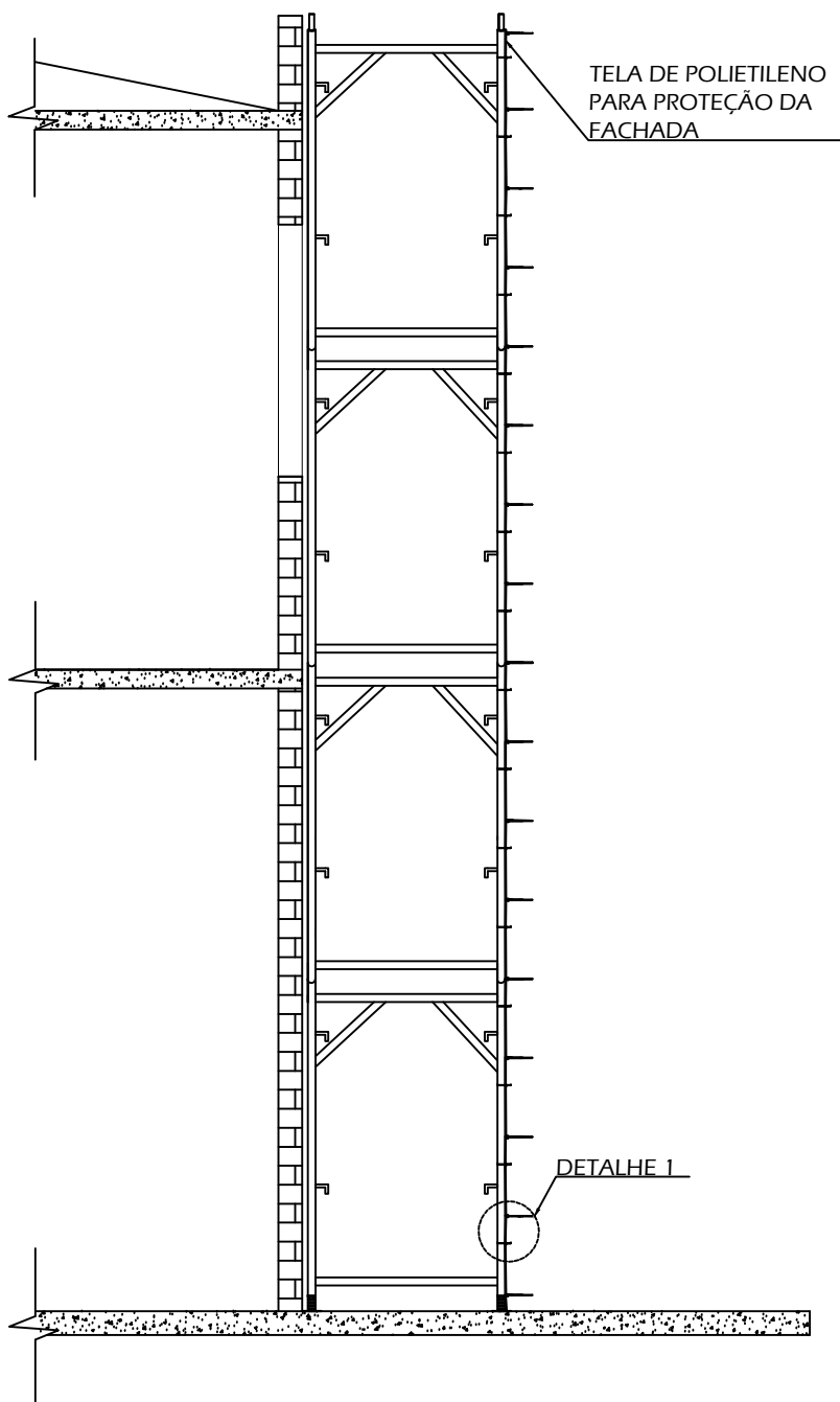
ELEVAÇÃO ESCALA 1/50
