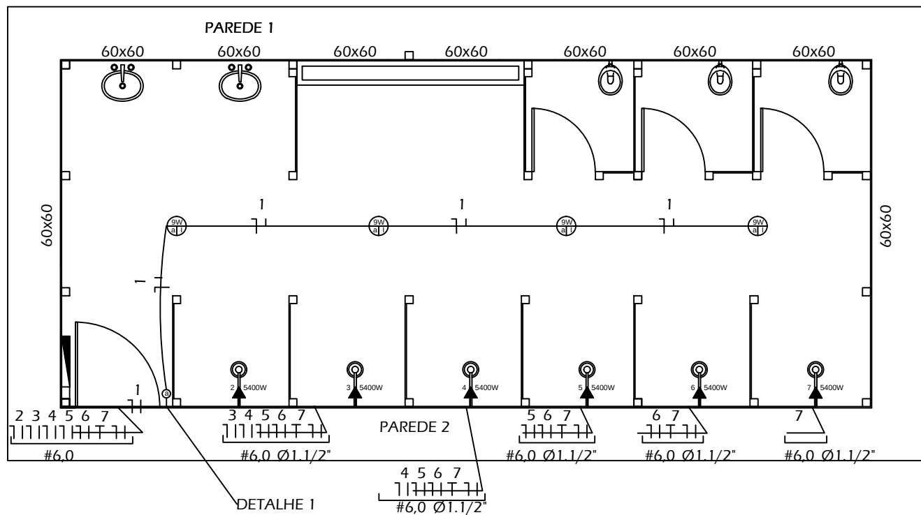
PLANTA - ELÉTRICO INSTALAÇÃO SANITÁRIA TIPO III
