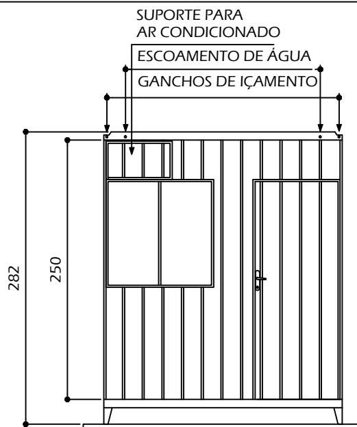
VISTA FRONTAL ESCALA 1/50
