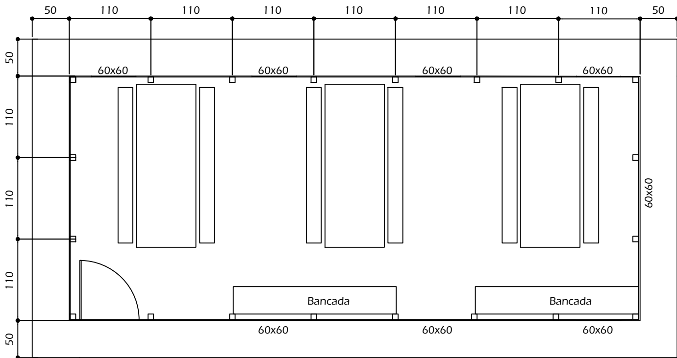
PLANTA - REFEITÓRIO TIPO II
