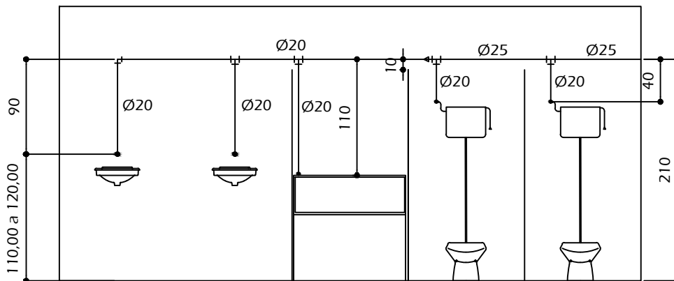
ÁGUA FRIA - PAREDE 1 - INSTALAÇÃO SANITÁRIA TIPO II ESCALA 1/50
