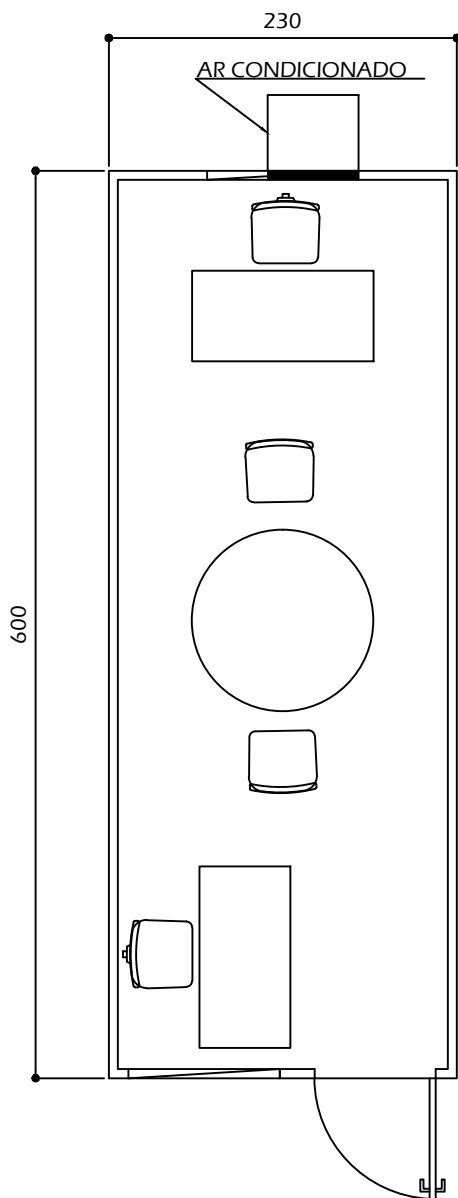
PLANTA ESCALA 1/50
