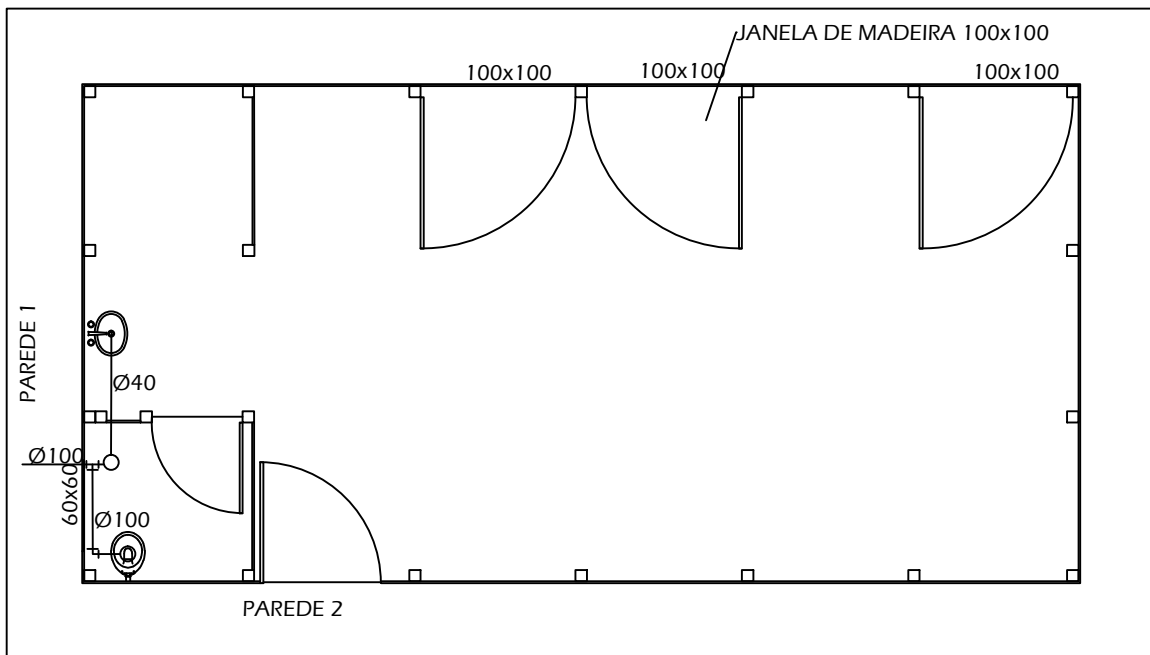
PLANTA - ESCRITÓRIO TIPO II
