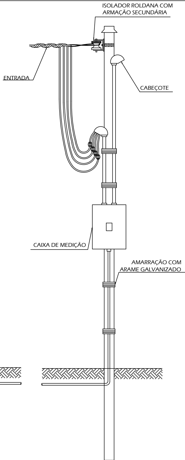
ELEVAÇÃO SEM ESCALA
