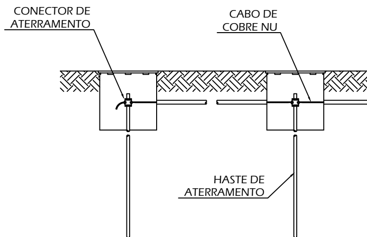
DETALHE ATERRAMENTO SEM ESCALA
