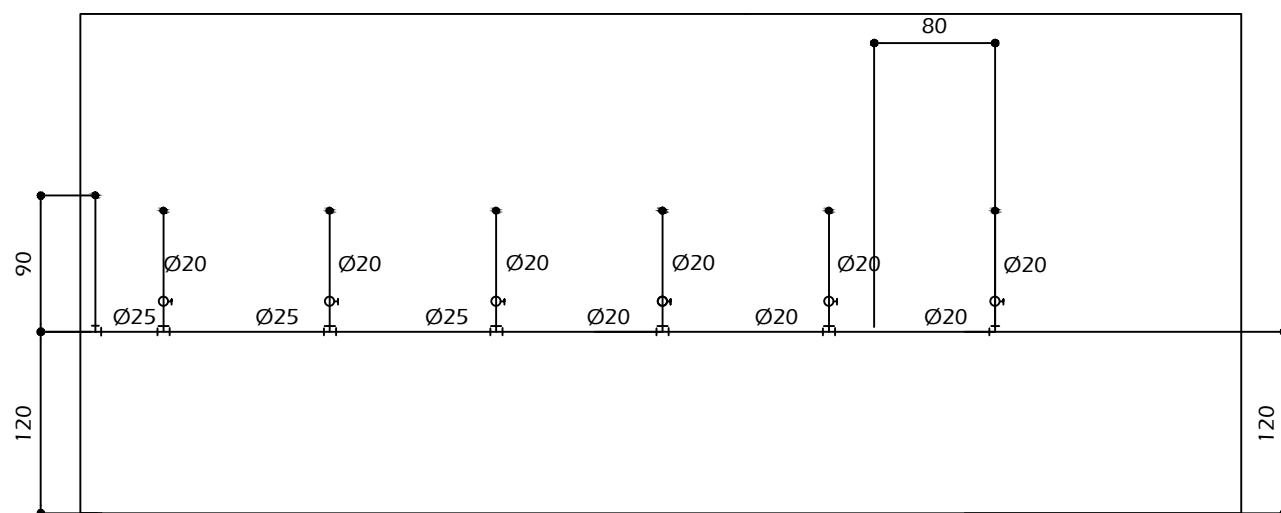
ÁGUA FRIA - PAREDE 2 - INSTALAÇÃO SANITÁRIA TIPO III ESCALA 1/50
