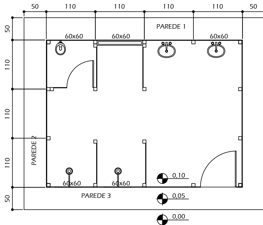
PLANTA - INSTALAÇÃO SANITÁRIA TIPO I ESCALA 1/50
