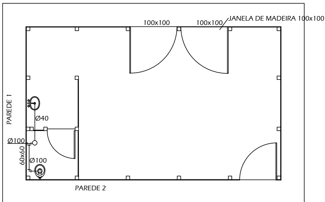
PLANTA - SANITÁRIO ESCRITÓRIO TIPO I ESCALA 1/50
