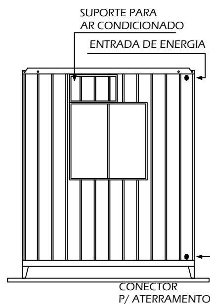
VISTA VISTA POSTERIOR ESCALA 1/50
