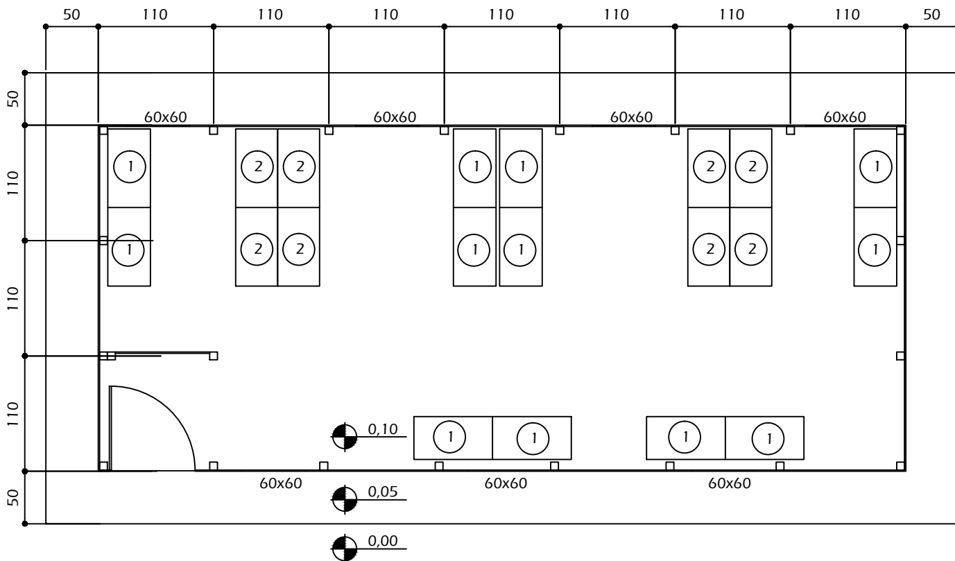
PLANTA - VESTIÁRIO TIPO I ESCALA 1/50
