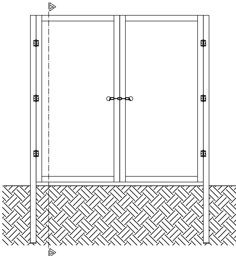
VISTA POSTERIOR ESCALA 1/25
