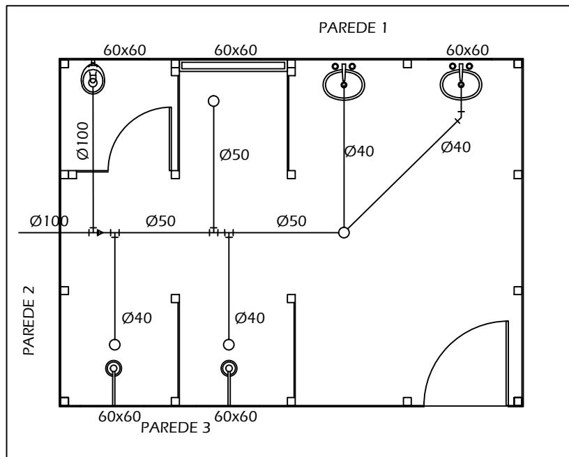
PLANTA - INSTALAÇÃO SANITÁRIA TIPO I
