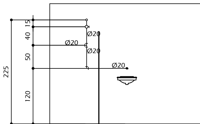
ÁGUA FRIA - PAREDE 1 - ESCRITÓRIO TIPO I ESCALA 1/50
