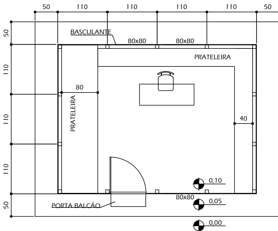
PLANTA - DEPÓSITO DE FERRAMENTAS TIPO I ESCALA 1/50
