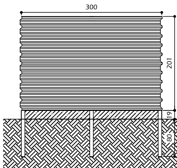
VISTA FRONTAL ESCALA 1/50
