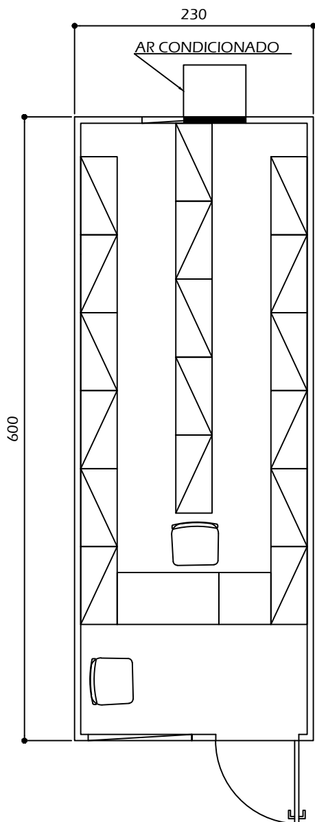
PLANTA ESCALA 1/50
