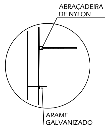
DETALHE 1 ESCALA 1/10
