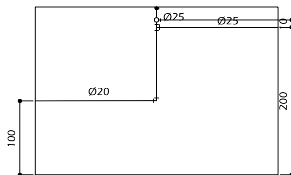
ÁGUA FRIA - PAREDE 1 - INSTALAÇÃO SANITÁRIA TIPO I
