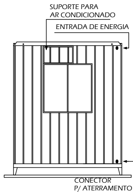
VISTA POSTERIOR ESCALA 1/50
