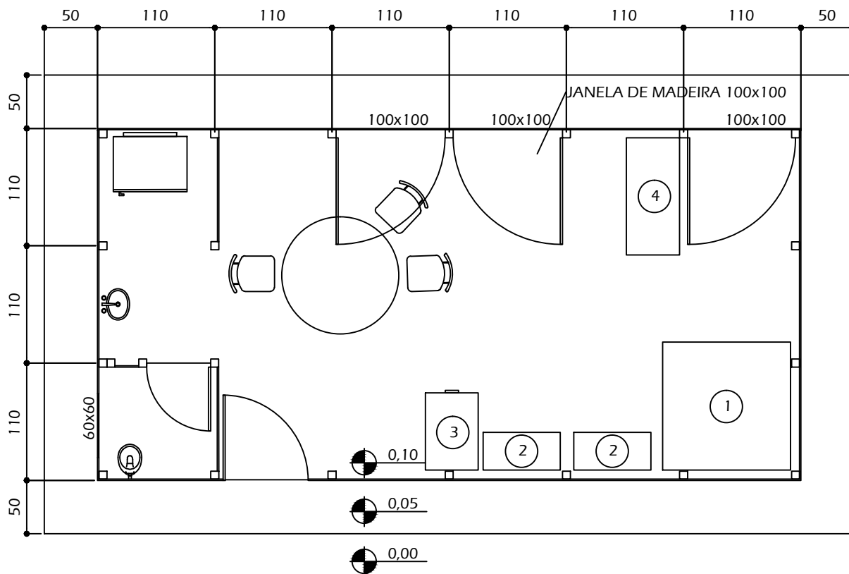
PLANTA - ESCRITÓRIO TIPO II ESCALA 1/50
