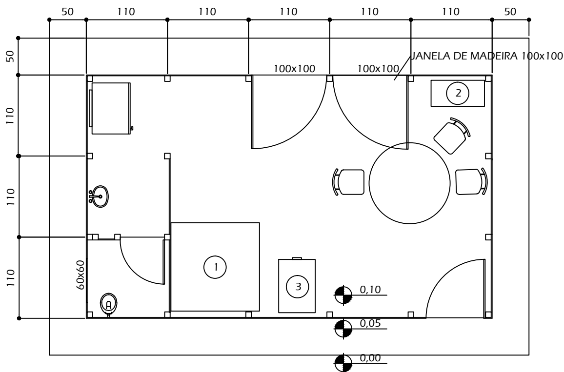
PLANTA - ESCRITÓRIO TIPO I ESCALA 1/50
