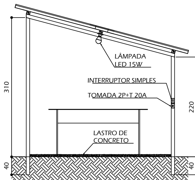
ELEVAÇÃO LATERAL
