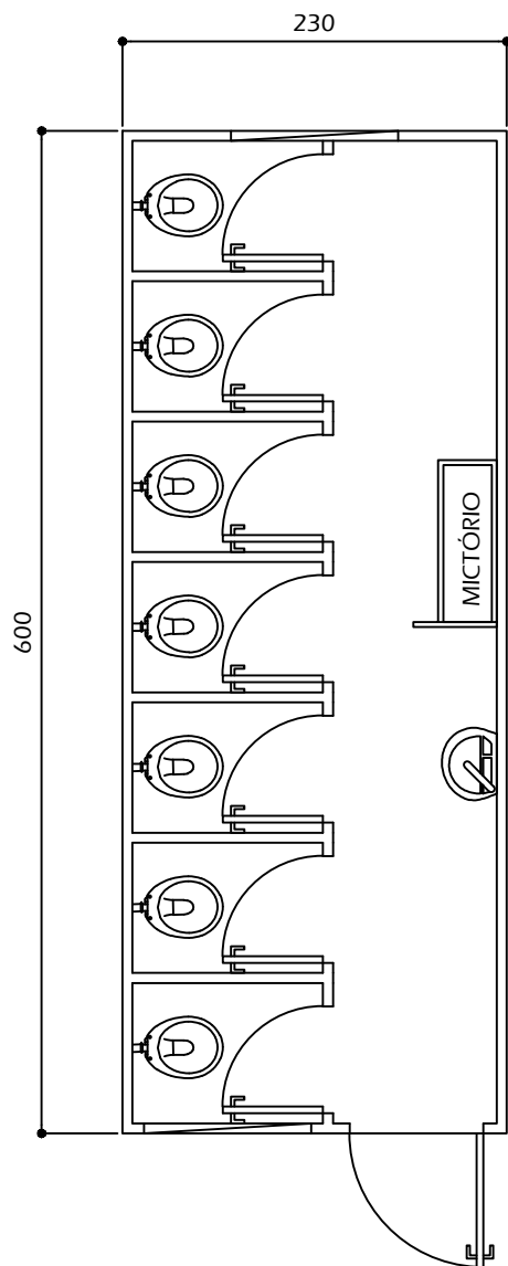
PLANTA ESCALA 1/50
